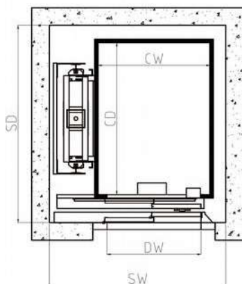
OLT - Oleodinamic 1:2
