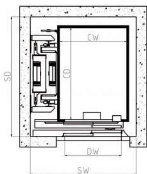
MRT - Side guide rail - 2:1
