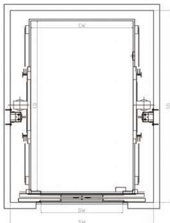
ODLD / ODLT Oleodinamic Double Side Piston
