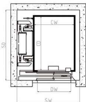
MRD - Side guide rail - 1:1
