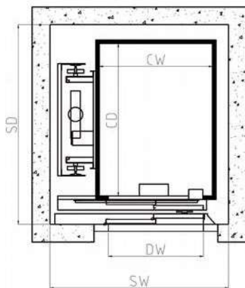
OLT - Oleodinamic 1:2
